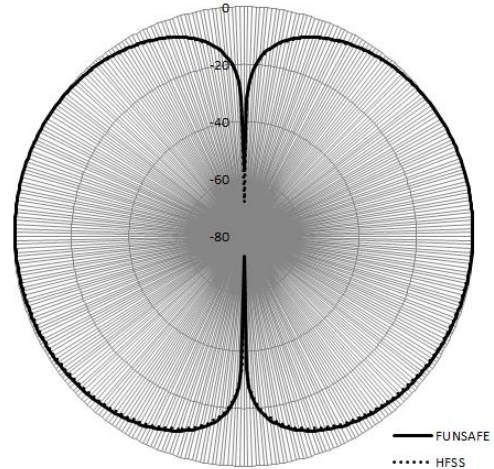
(b) H-plane
