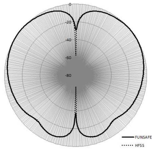
(b) H-plane
